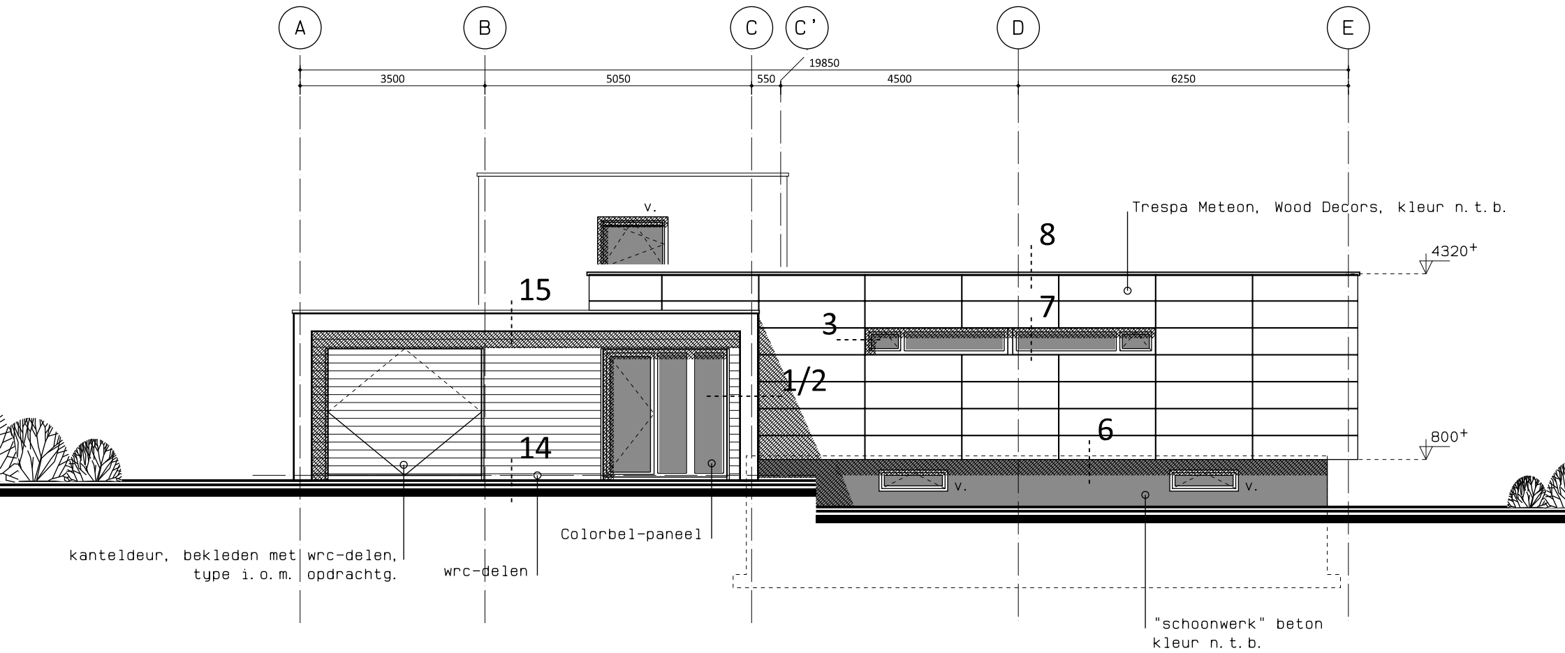
Noord-westgevel
