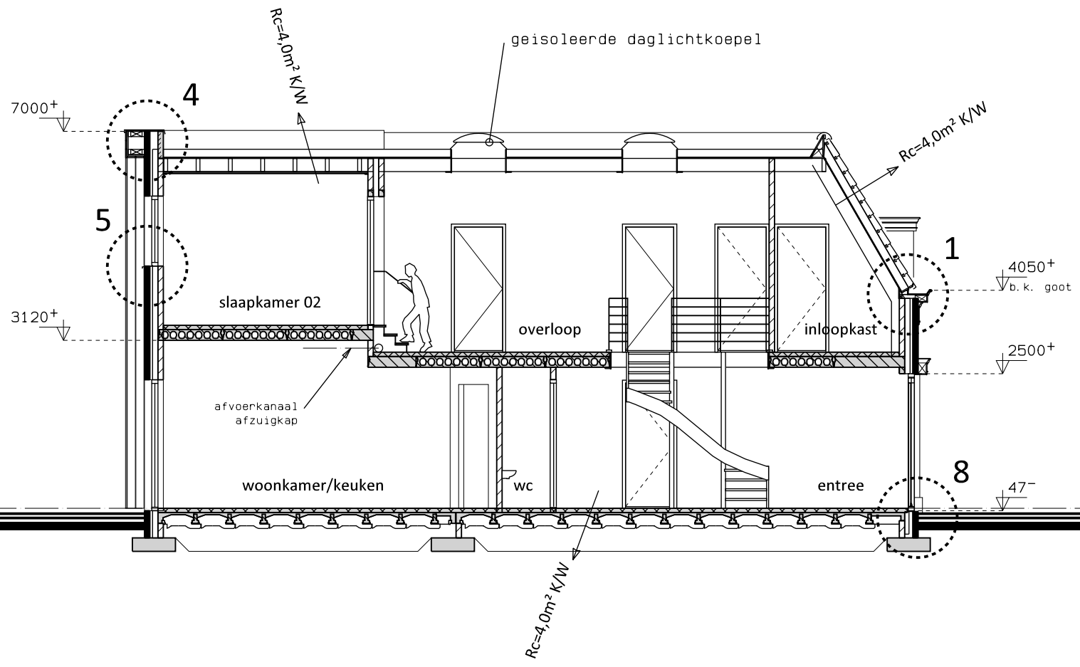
Doorsnede A-A
