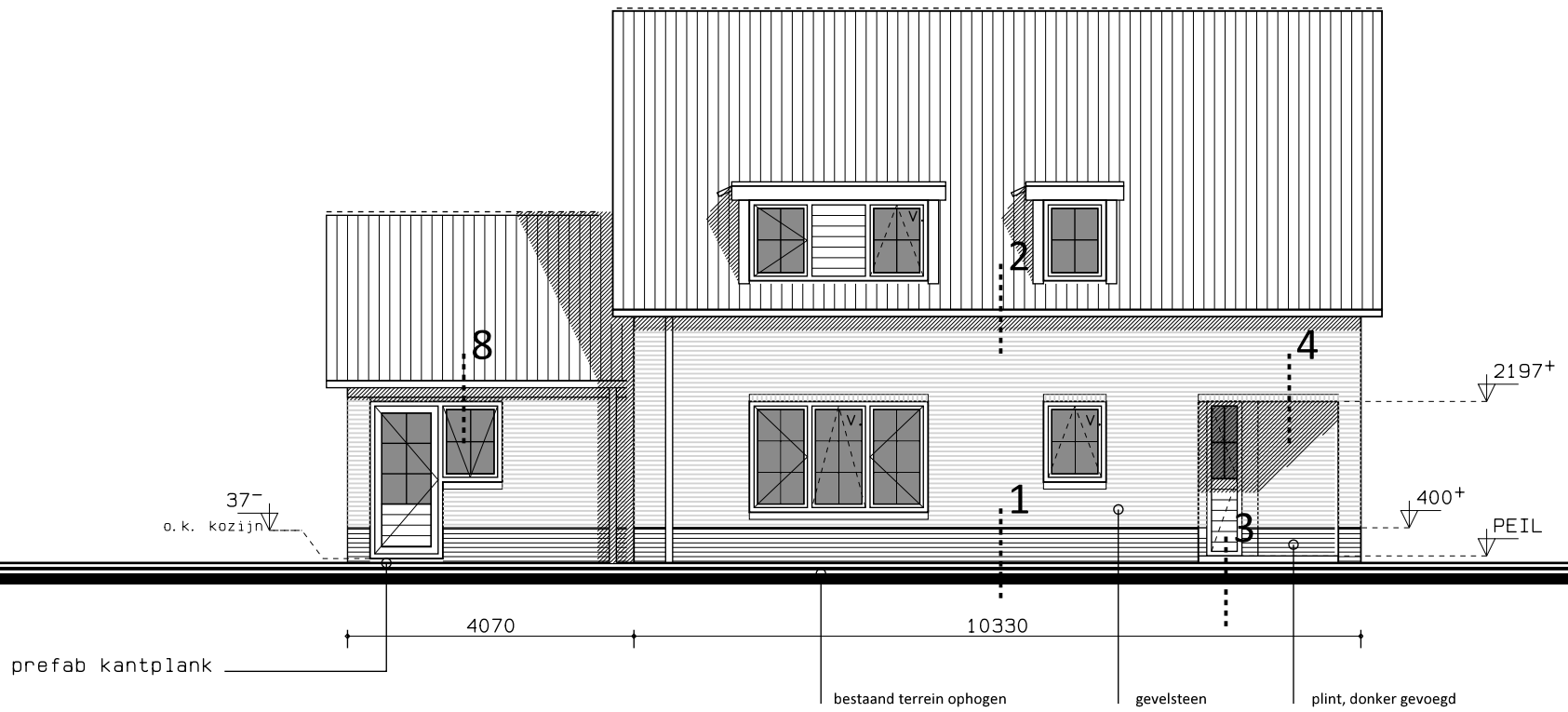
Noord-westgevel
